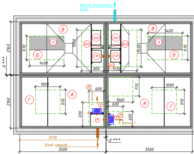
Схема станции
