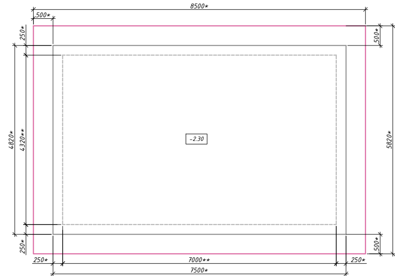
План котлована с плитой
